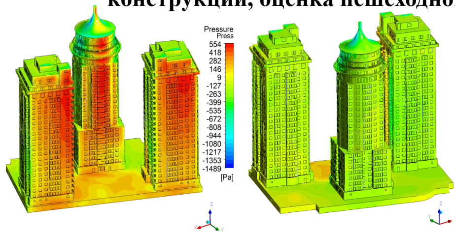
Средние давления на несущие конструкции (Па). Угол атаки ветра 0^\circ
