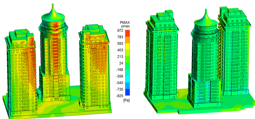
Максимальные давления (Па) на фасадные конструкции для угла атаки ветра 0^\circ . Максимальное значение 972 Па, минимальное -925 Па
