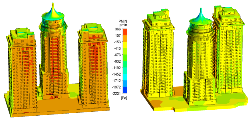
Минимальные давления (Па) на фасадные конструкции для угла атаки ветра 0^\circ . Максимальное значение 366 Па, минимальное -2231 Па
