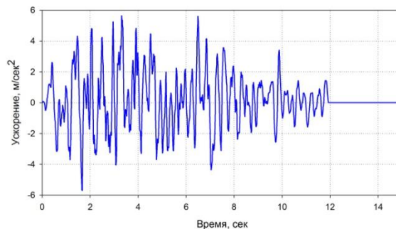
Акселерограмма, соответствующая МРЗ
