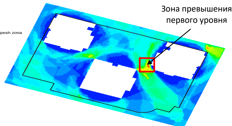
1-й уровень пешеходной комфортности – повторяемость скорости ветра в порывах 6 м/с (час/год), коэффициент обеспеченности \Theta = 2 . Допустимая величина – 1000 час
