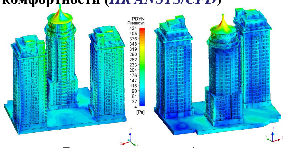
Пульсационная составляющая давления на несущие конструкции (Па). Угол атаки ветра 0^\circ
