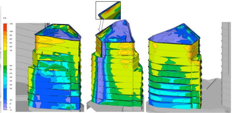
Рисунок 5 – ЖК «Акватория», Ленинградское ш., г. Москва
