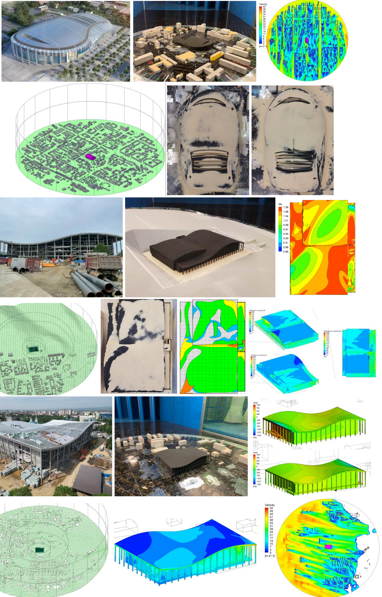
Рисунок 19 – Ледовая арена, универсальный спортивный комплекс и центр водных видов спорта, г. Южно-Сахалинск
