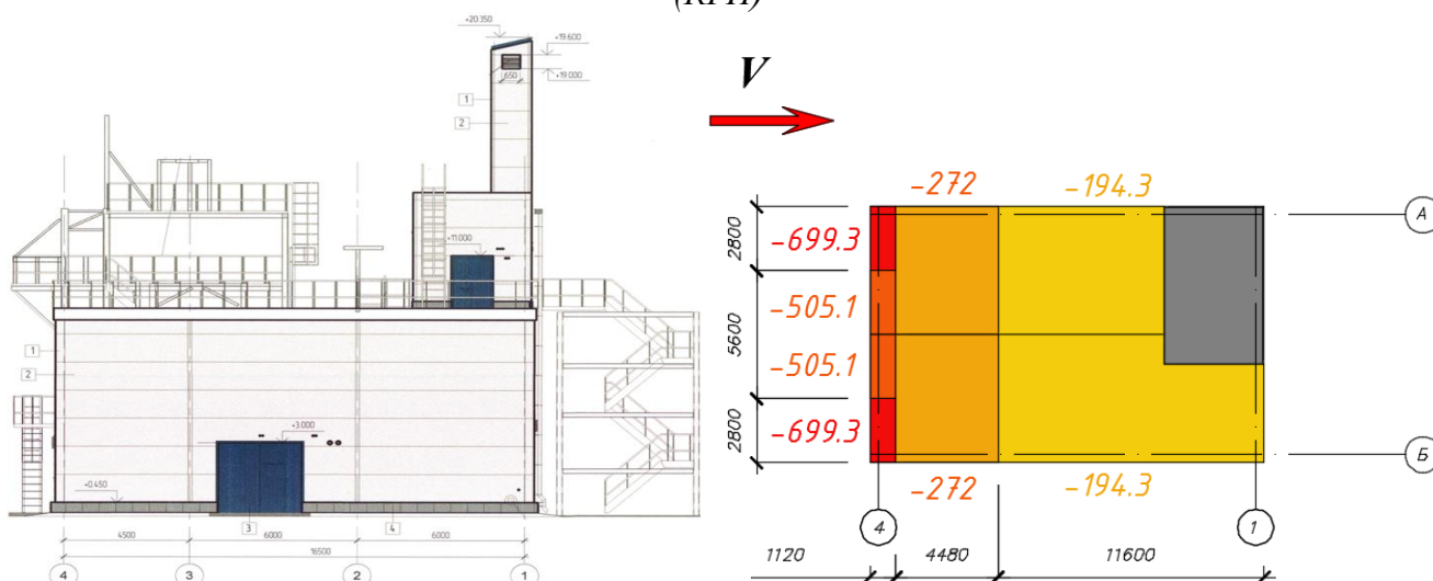
Технологические объекты АО «Газпромнефть-ОМПЗ, г. Омск Рисунок 32 – Расчеты объектов добывающей промышленности
