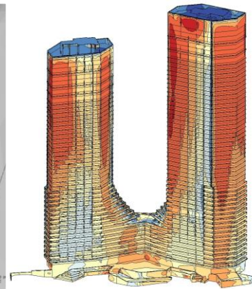
Рисунок 10 – ЖК «JOIS», 3-й Силикатный проезд, г. Москва
