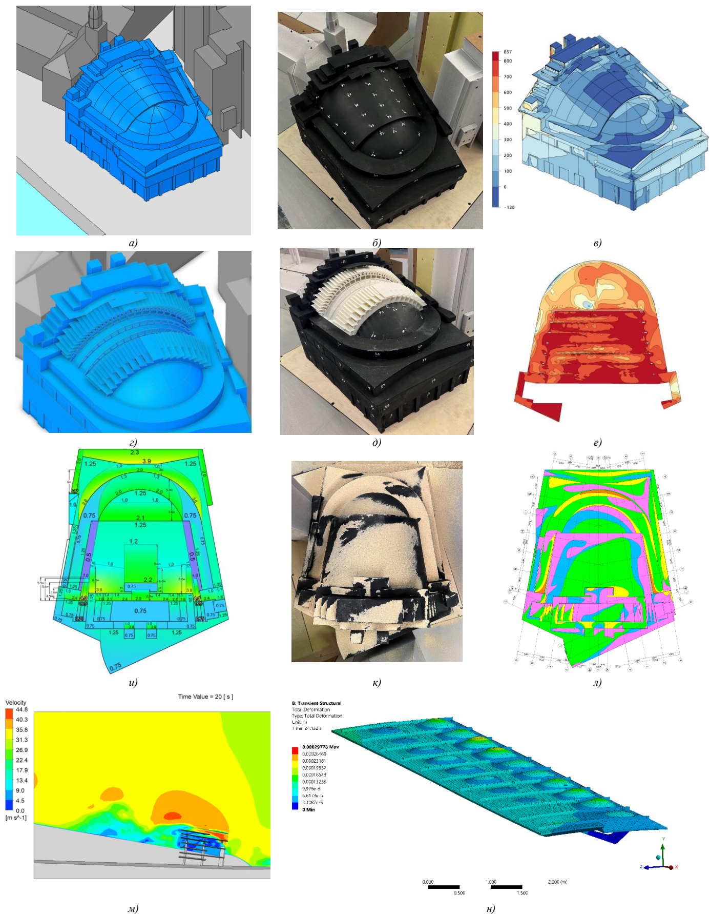
Рисунок 28 – Реконструкция кинотеатра «Ударник», г. Москва: а-в) модель с закрытыми панелями г-е) модель с открытыми панелями и-л) расчеты и эксперименты на определение снеговых нагрузок, м-н) расчеты эффектов аэроупругости панелей покрытия
