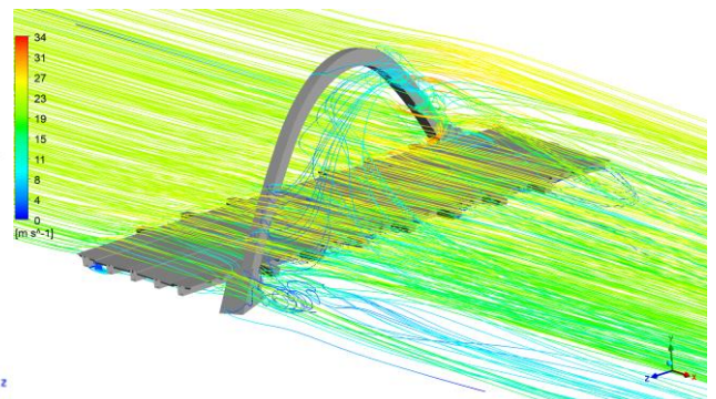
Рисунок 36 – Автодорожный мост через залив реки Москвы на проезде пр. 7101 территории Рублево-Архангельское района Кунцево, г. Москва
