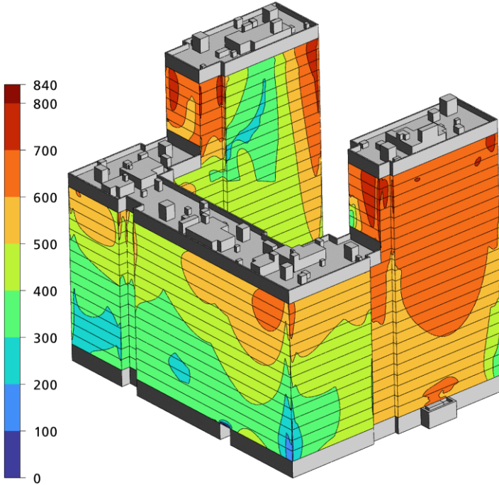
Рисунок 38 – Численное моделирование ветровых нагрузок, разработка методики нелинейного расчета для трехслойных самонесущих навесных панелей серии НП1.1 и оценках их несущей способности
