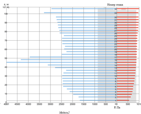
Рисунок 11 – ЖК по программе реновации, ул. Подвойского, г. Москва
