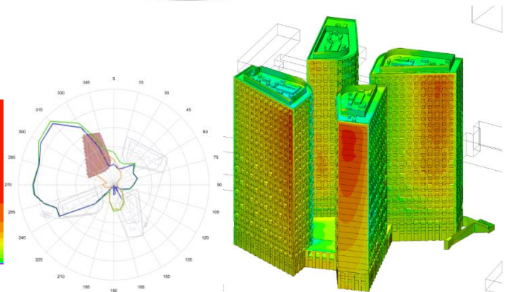
Рисунок 4 – ЖК «Level Нагатинская», Нагатинская наб., г. Москва
