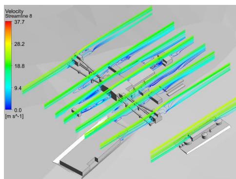
Рисунок 29 Расчеты сооружений ПАО «НЛМК», г. Липецк
