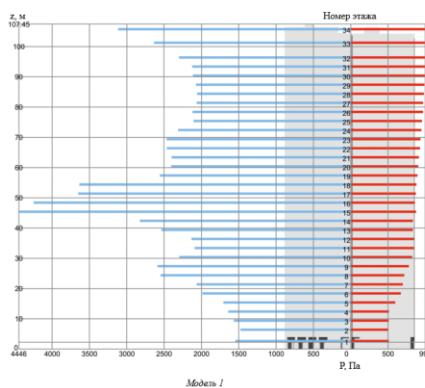
Рисунок 11 – ЖК по программе реновации, ул. Подвойского, г. Москва
