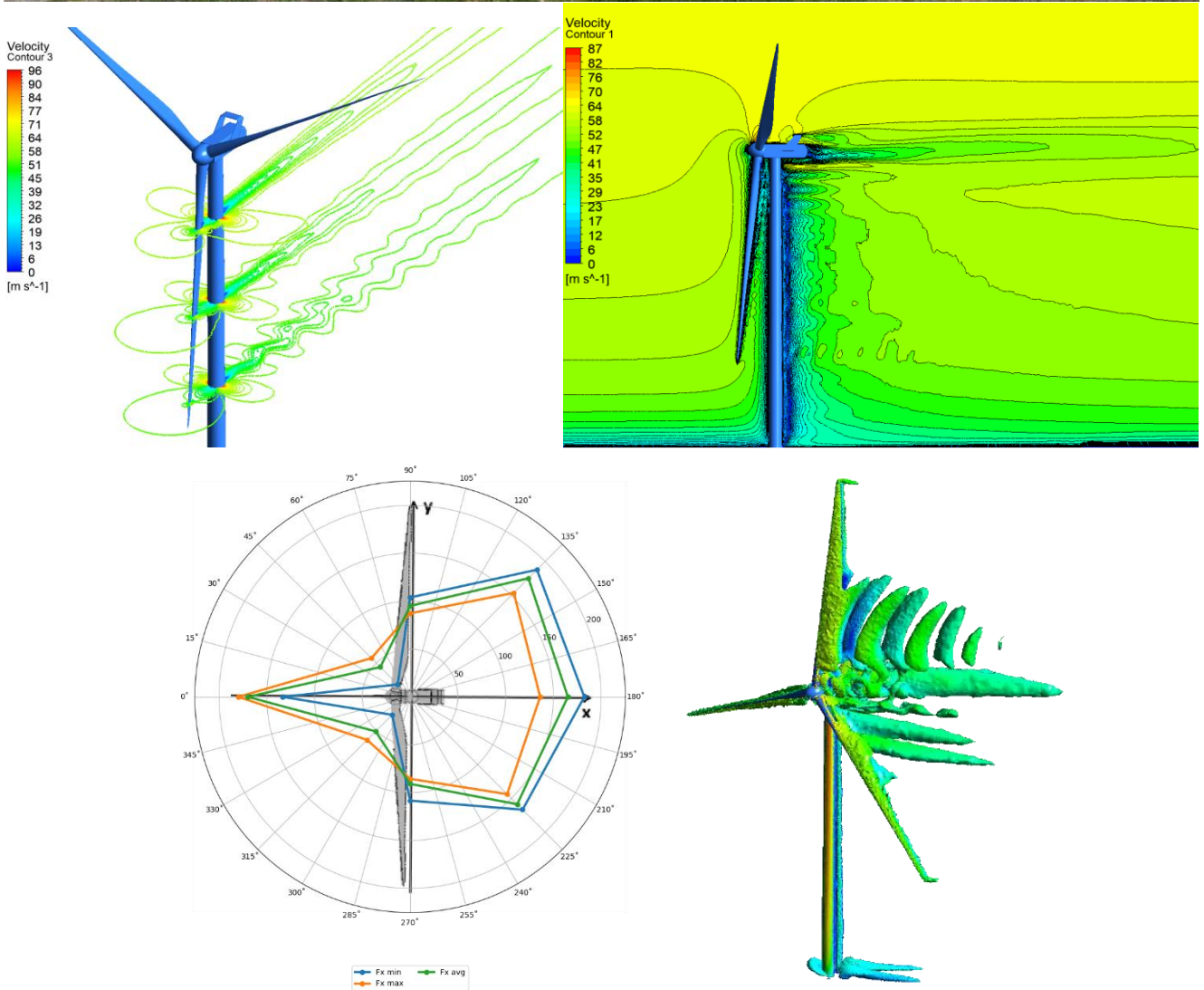
Рисунок 37 – Расчеты ветровых энергоустановок (5 объектов в Ульяновской и Ростовской областях)
