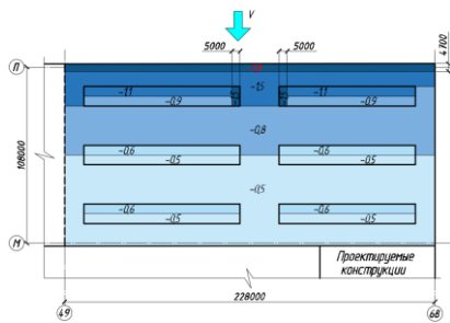
Рисунок 29 Расчеты сооружений ПАО «НЛМК», г. Липецк
