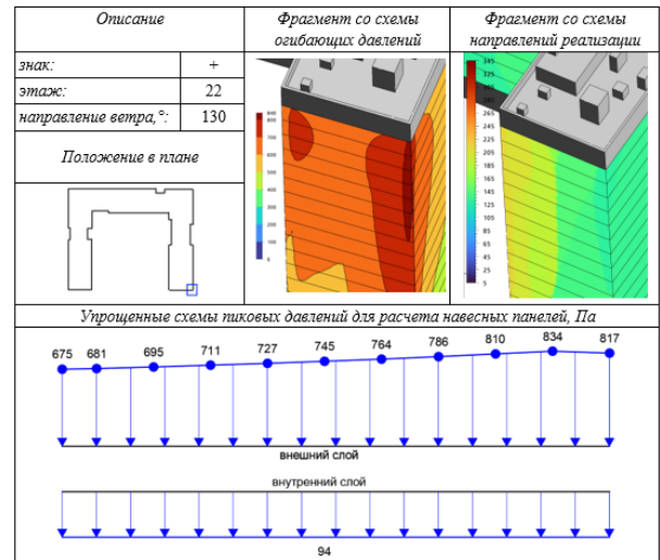
Рисунок 38 – Численное моделирование ветровых нагрузок, разработка методики нелинейного расчета для трехслойных самонесущих навесных панелей серии НП1.1 и оценках их несущей способности
