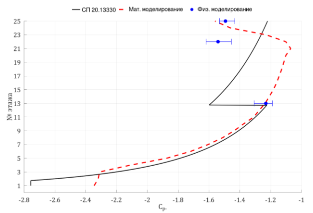
Пиковые отрицательные аэродинамические коэффициенты C_{p-} для окон
