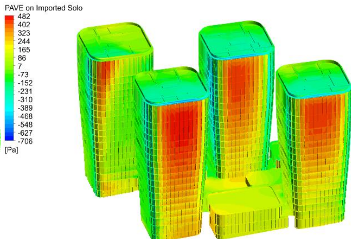
Рисунок 6 – ЖК «Sky View», ул. Дружинниковская, г. Москва
