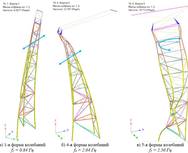
Рисунок 35 – Стела «Город трудовой доблести», г. Екатеринбург
