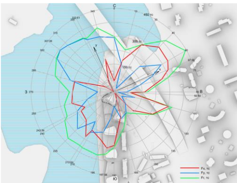
Рисунок 5 – ЖК «Акватория», Ленинградское ш., г. Москва
