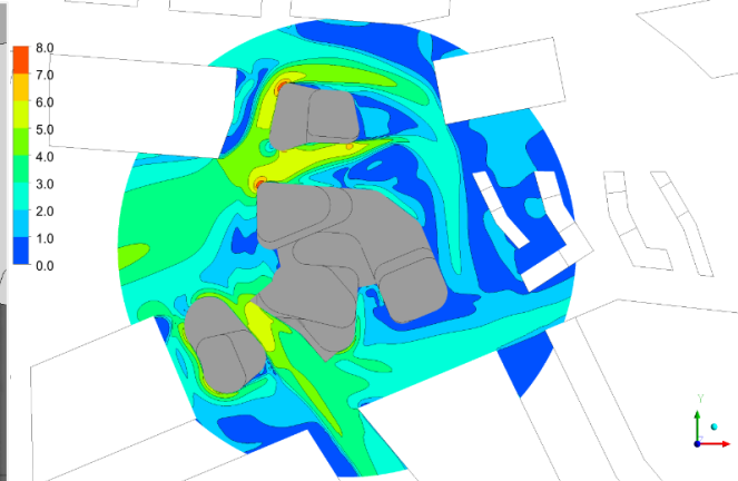
Рисунок 13 – Офисно-деловой центр в поселке Рублево-Архангельское, г. Москва
