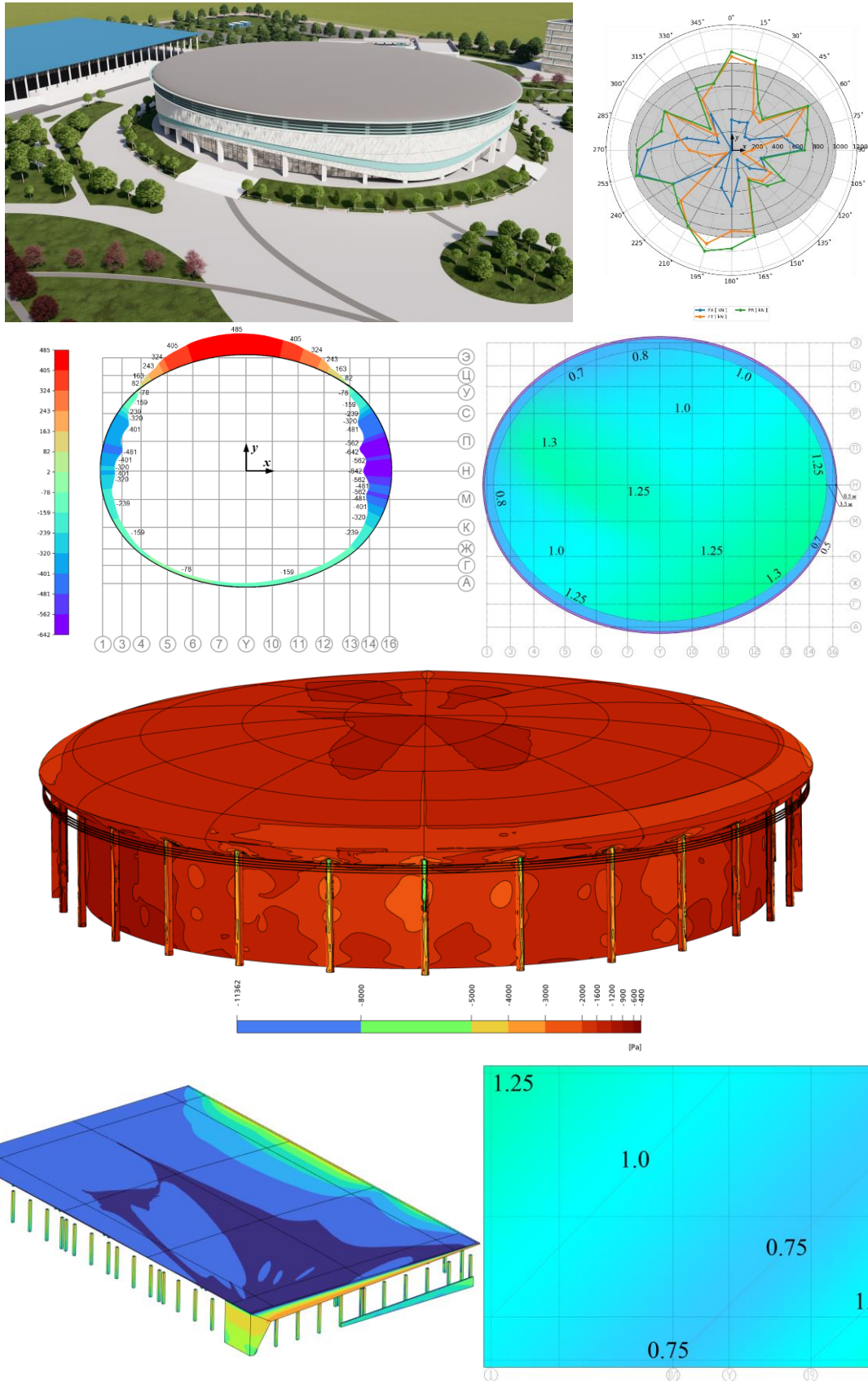
Рисунок 21 – Центр велосипедного спорта - здание Велодрома и Навес трассы BMX, г. Майкоп
