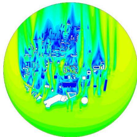
Рисунок 2 – ЖК «Прайм парк», г. Москва
