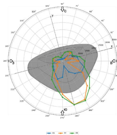
Рисунок 23 – МФК гостиничный комплекс, г. Алушта
