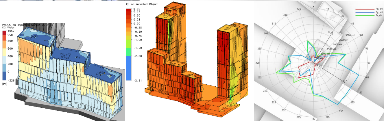
Рисунок 1 – МФК на ул. Архитектора Власова, г. Москва
